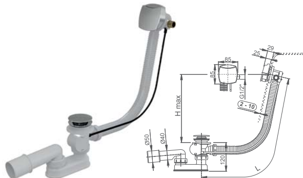
■ sifón vaňový s napúšťaním prepadom
